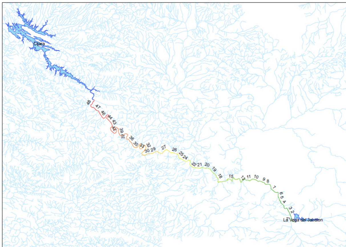
Ilustración 6. Distancia hipotética que recorrerían las larvas de mejillón cebra por hora en el tramo del cauce comprendido entre los embalses de La Vega del Jabalón y Cijara.
