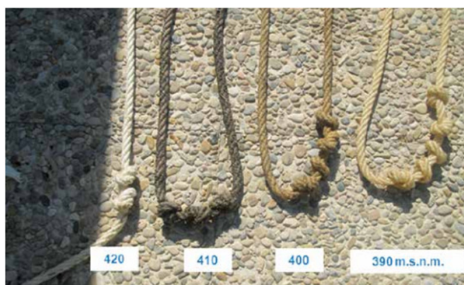
Ilustración 22. Muestra del método de identificación de cotas por nudos en los testigos colocados en el Embalse de Iznájar. Fuente: Confederación Hidrográfica del Guadalquivir
