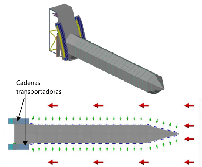
Ilustración 27. Detalles del filtro de final del canal. Fuente: Filtros Palacios, S.L.
